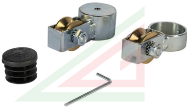
Doppie carrucole per aste Ø 32 mm Dual pulley for Ø 32 mm flagpole
