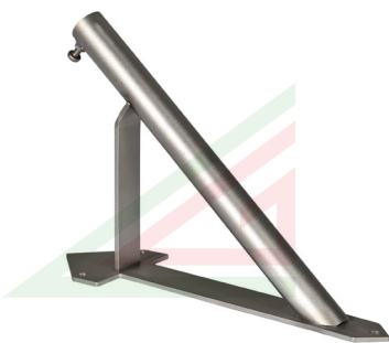
Supporto a muro, 1 posto per aste Ø 25 mm Wall bracket, 1 place for Ø 25 mm flagpole
